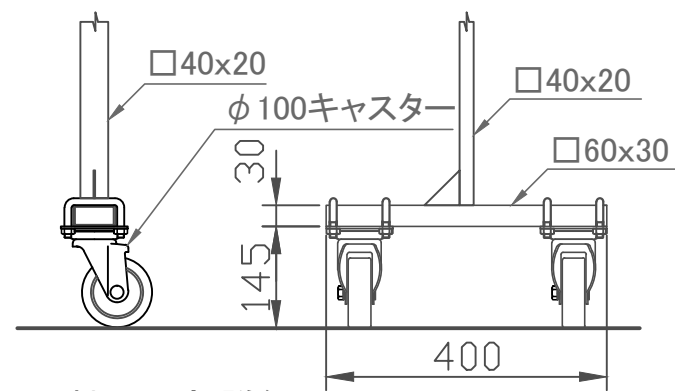
軸足下部詳細
