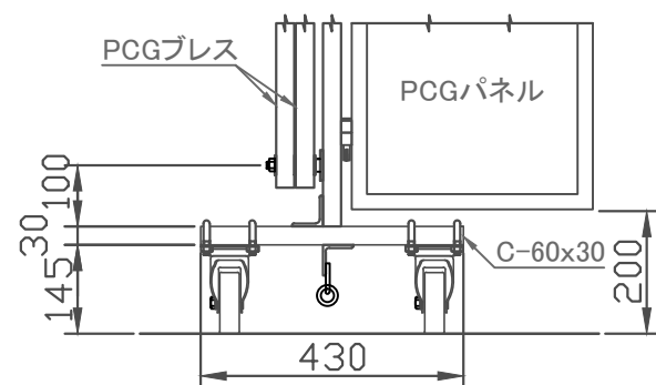
走行棒下部詳細
