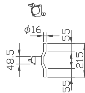
丁番クランプ詳細
