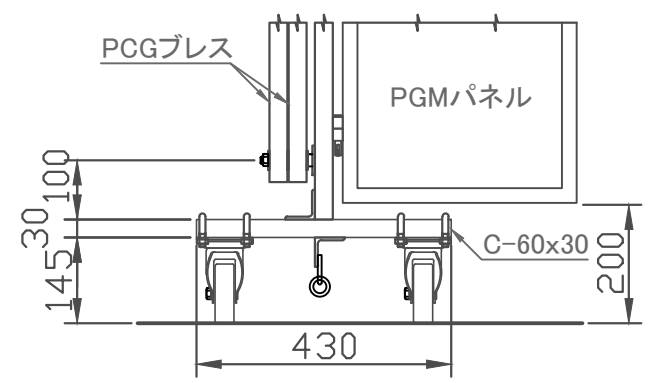
走行棒下部詳細
