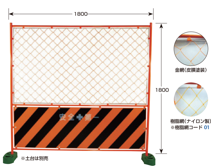
ガードフェンス トラ 1800×1800mm 8kg B-031 B-031-01
